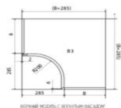
ВЕРХНИЙ ИЗОДЪЕЛ С ВОЗДУШНЫМ ФАСАДОМ
