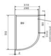
НИЖНИЙ ИЗОДЪЕЛ С ПЛЫТНЫМ ФАСАДОМ
