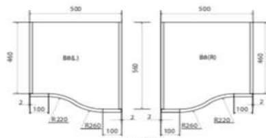
НИЖНИЙ ИЗОДЪЕЛ С С - ОБРАЗНЫМ ФАСАДОМ
