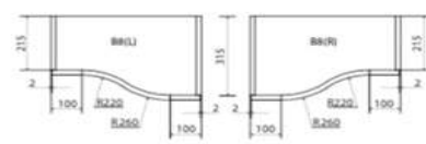
ВЕРХНИЙ ИЗОДЪЕЛ С С - ОБРАЗНЫМ ФАСАДОМ
