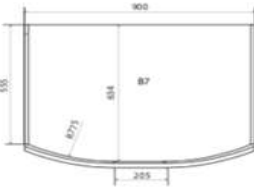
НИЖНИЙ МОДУЛЬ С ПУГЛЫМ ФАСАДОМ КАСТРЮЛЬНИЦА
