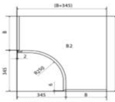
НИЖНИЙ МОДУЛЬ С ВОГУЛЫМ ФАСАДОМ
