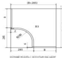
ВЕРХНИЙ ПРОФИЛЬ С ВОГНУТЫМ ФАСАДОМ
