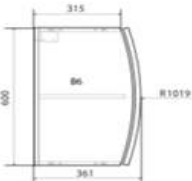
ВЕРНИЙ МОДУЛЬ С ПУГЛЫМ ФАСАДОМ
