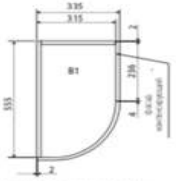
НИЖНИЙ МОДУЛЬ С ПУГЛЫМ ФАСАДОМ
