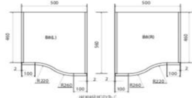
НИЖНИЙ ПРОФИЛЬ С S-ОБРАЗНЫМ ФАСАДОМ
