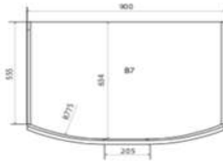
НИЖНИЙ ПРОФИЛЬ С ПУХТЫМ ФАСАДОМ ИМАКСПРЕДПРОФИЛЕМ
