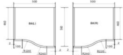
НИЖНИЙ МОДУЛЬ С С - ОБРАЗНЫМ ФАСАДОМ
