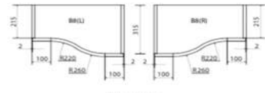
ВЕРХНИЙ ПРОФИЛЬ С S-ОБРАЗНЫМ ФАСАДОМ
