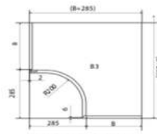
ВЕРНИЙ МОДУЛЬ С ВОГУЛЫМ ФАСАДОМ
